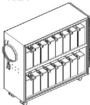
MÓDULO BATERIAS GRANDE SEL. 16 x 17Ah 192V
